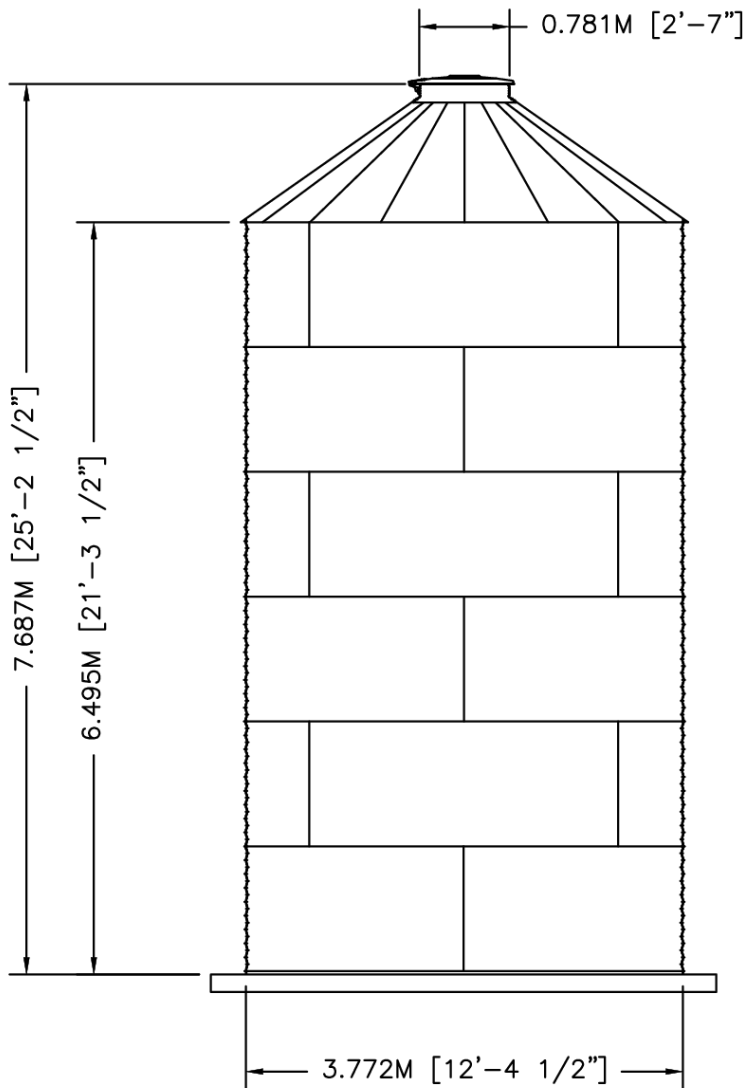
ELEVATION
